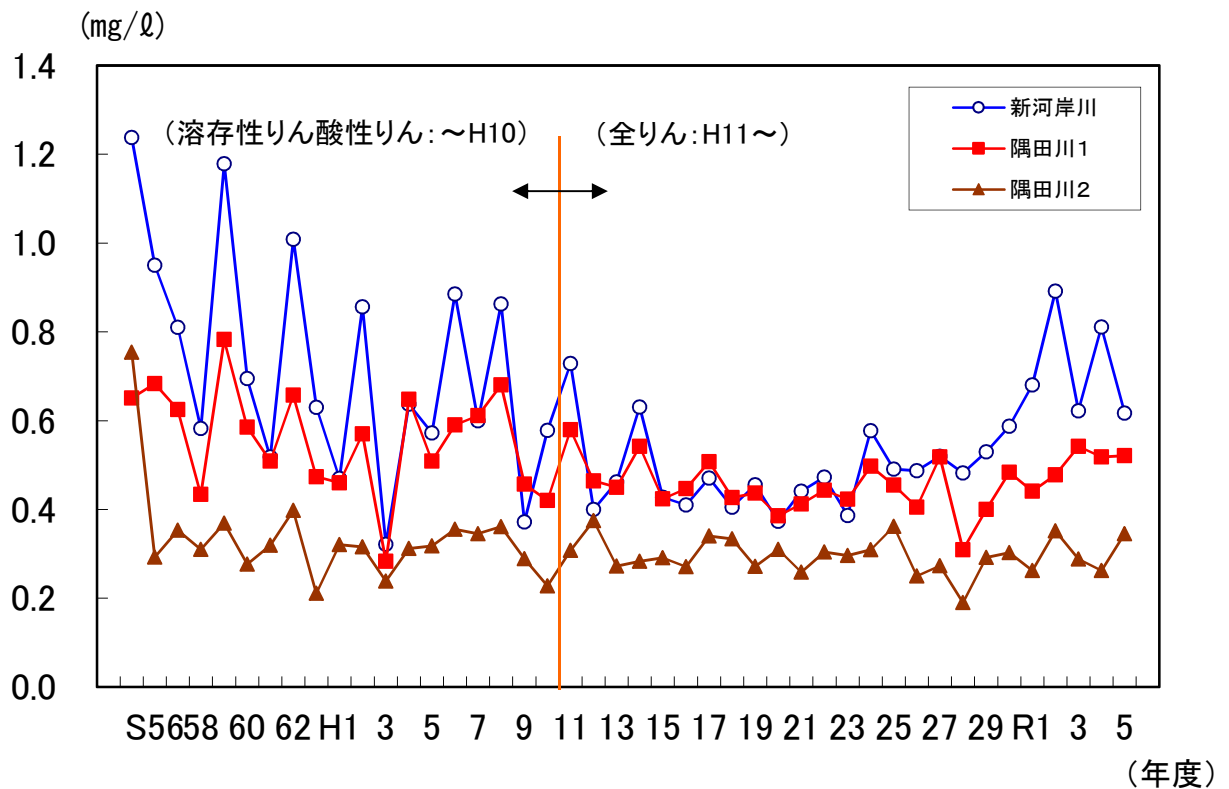
図18 新河岸川・隅田川の全りん・溶存性りん酸性りん経年変化(拡大図)
