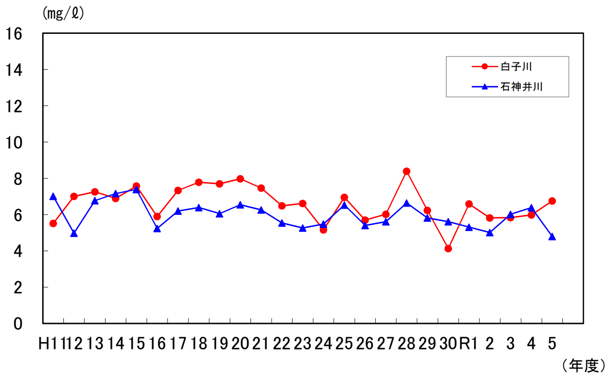
図15 白子川・石神井川の全窒素(T-N)経年変化
