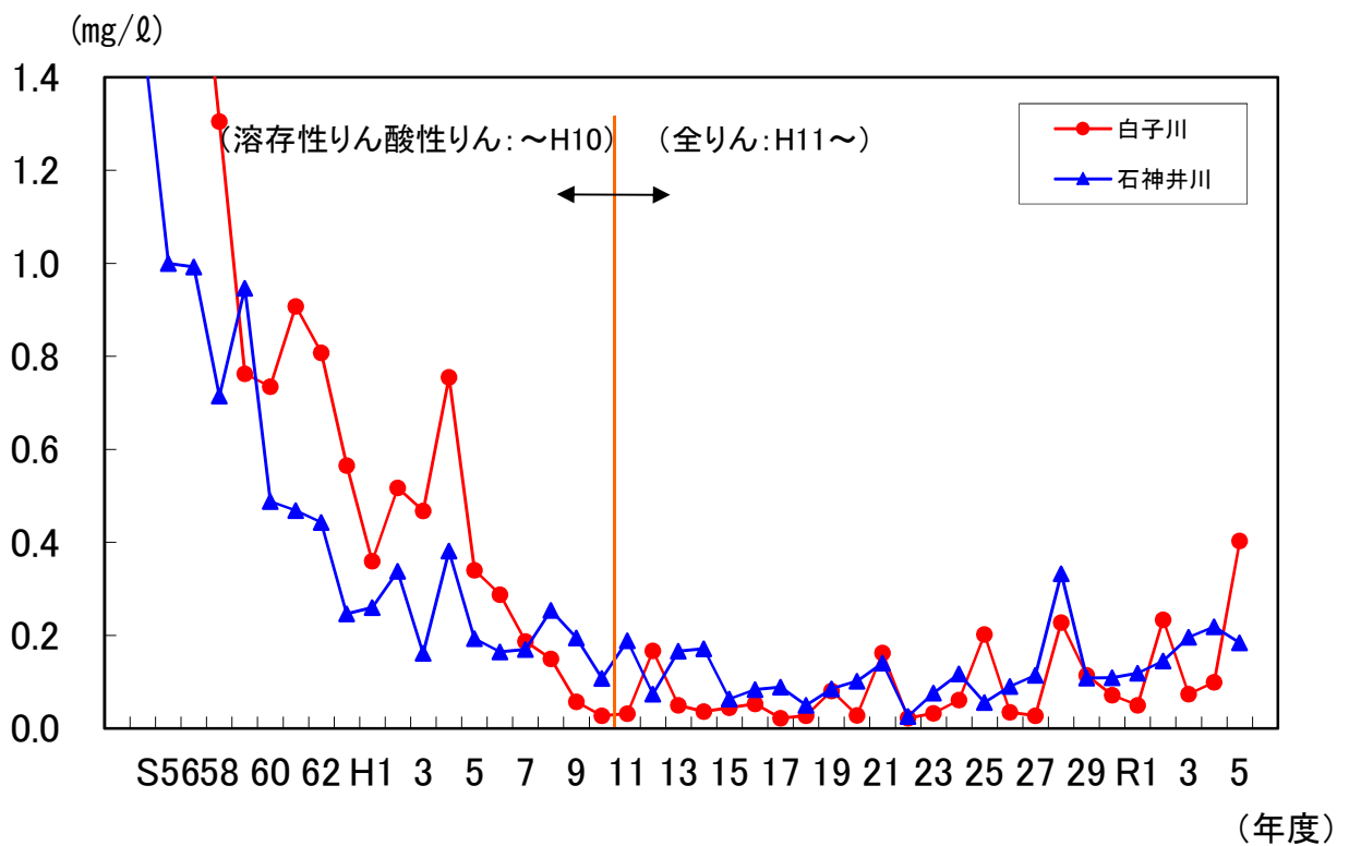
図19 白子川・石神井川の全りん・溶存性りん酸性りん経年変化(拡大図)
