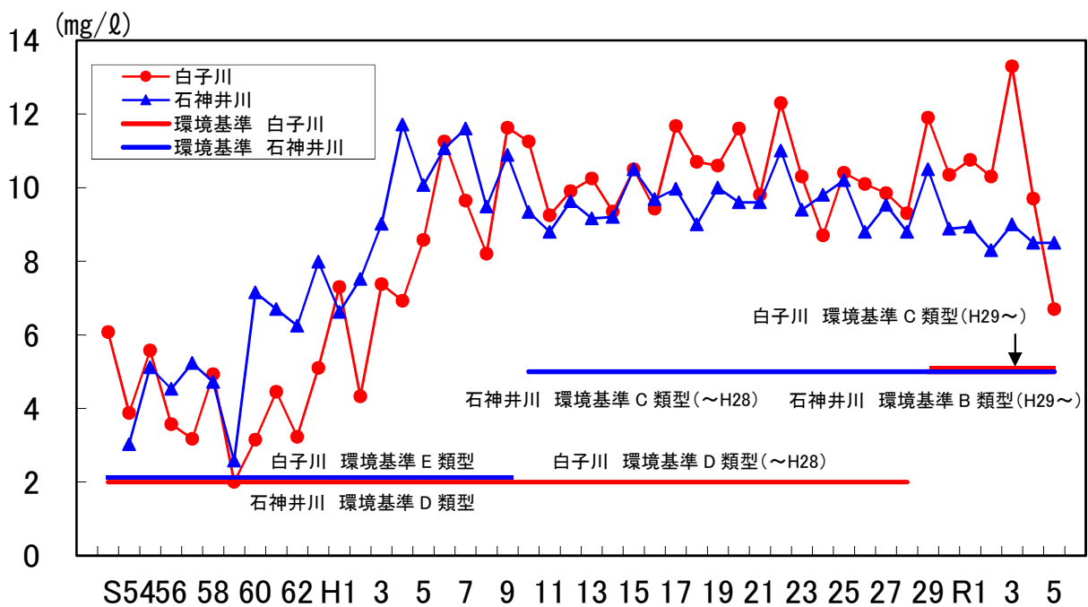
図10 白子川・石神井川の溶存酸素量(DO)経年変化 (年度)
