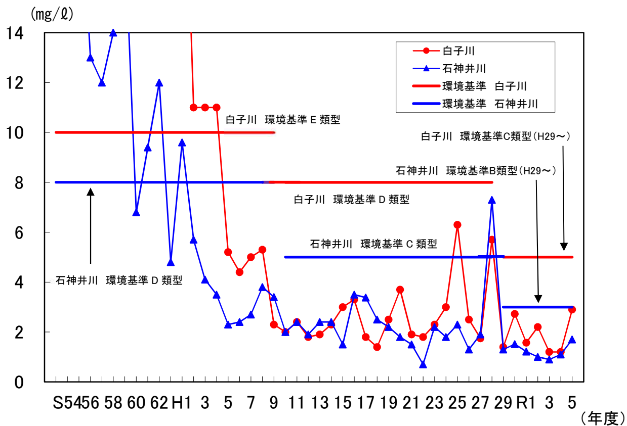
図13 白子川・石神井川の生物化学的酸素要求量(BOD)経年変化 (拡大図)
