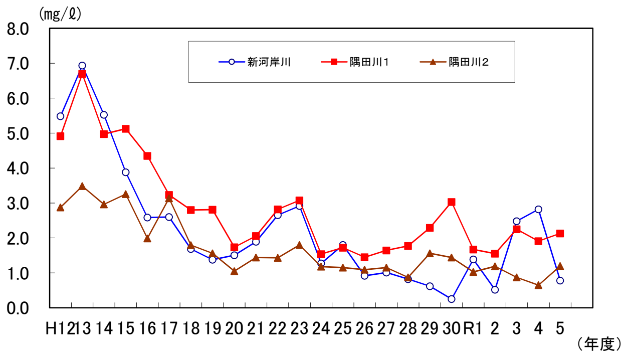
図20 新河岸川・隅田川のアンモニア性窒素( \text{NH}_4^+\text{-N} )経年変化
