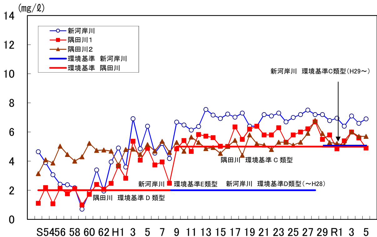
図9 新河岸川・隅田川の溶存酸素量(DO)経年変化 (年度)
