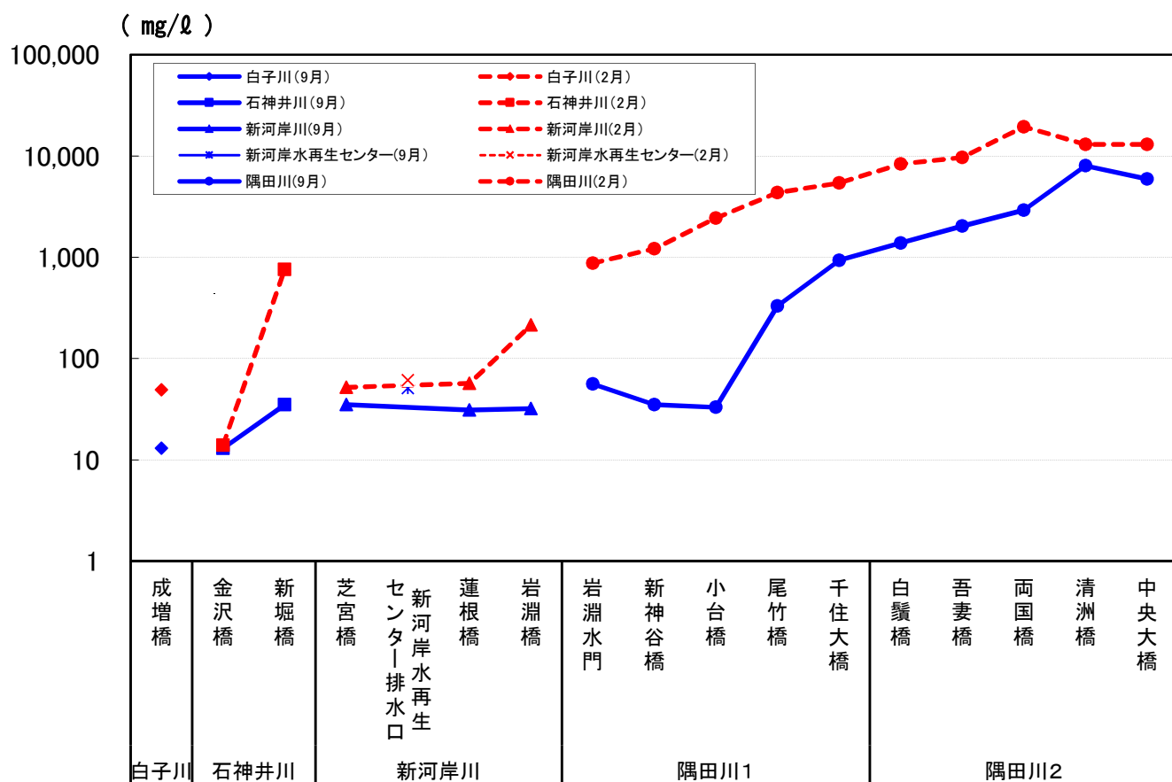
図5 塩化物イオン(Cl⁻)縦断変化
