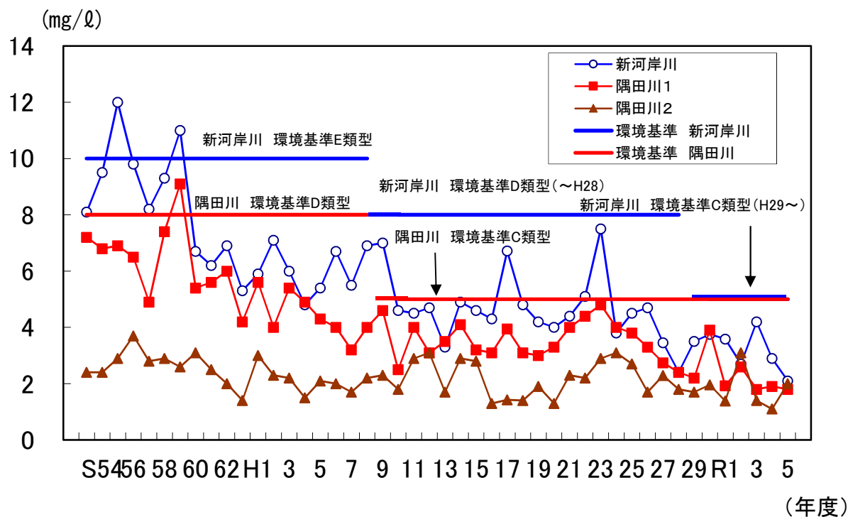
図11 新河岸川・偶田川の生物化学的酸素要求量(BOD)経年変化
