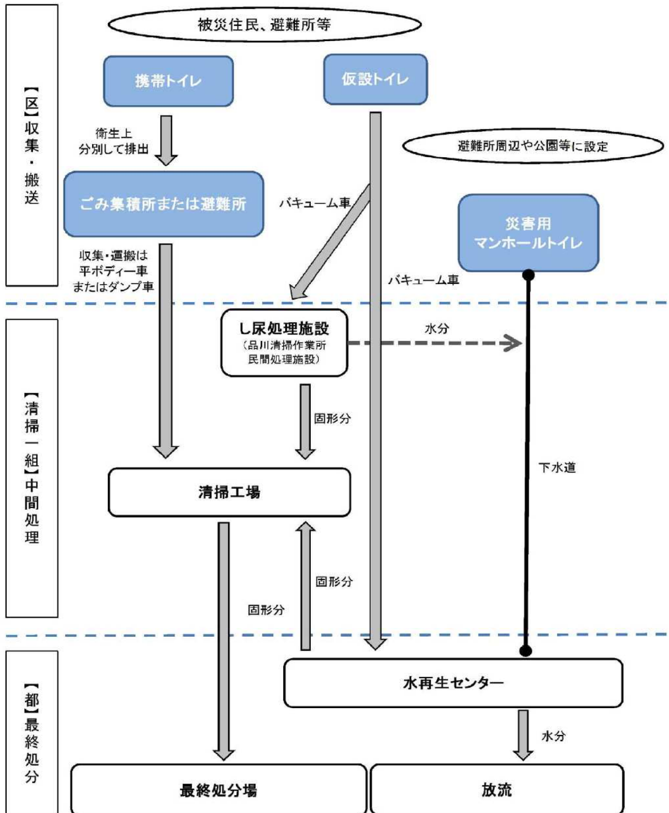
図5 し尿の標準処理フロー
