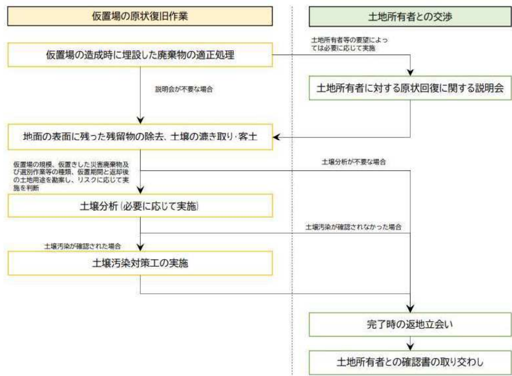
図 16 一次仮置場の原状回復フロー
