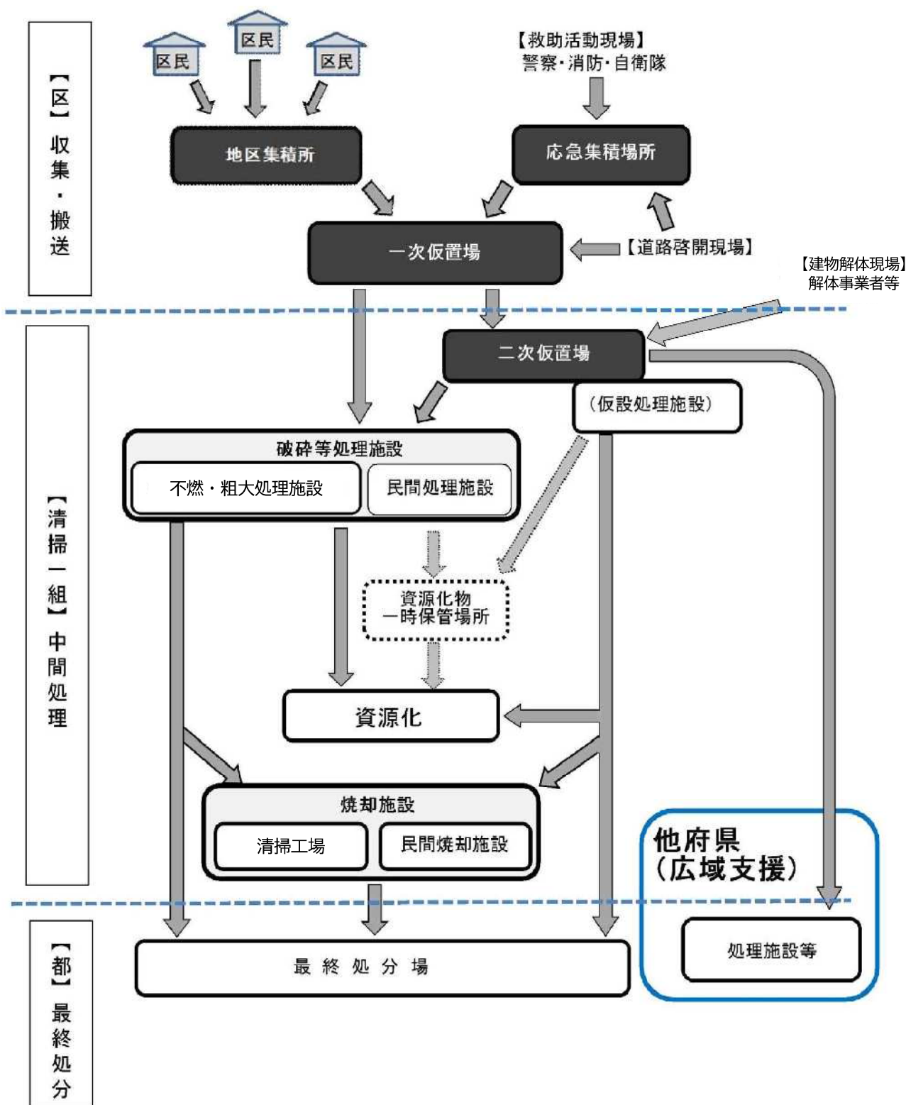
図2 がれき等の標準処理フロー
