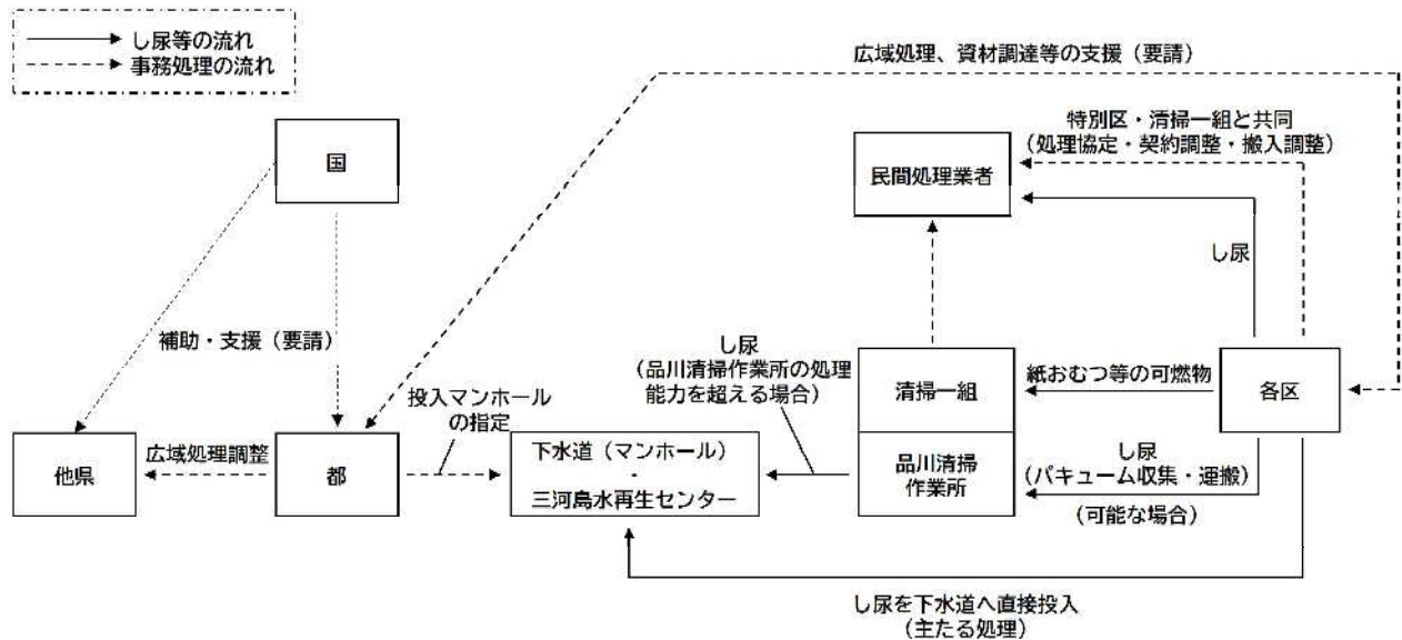
図9 し尿処理の基本フロー図
