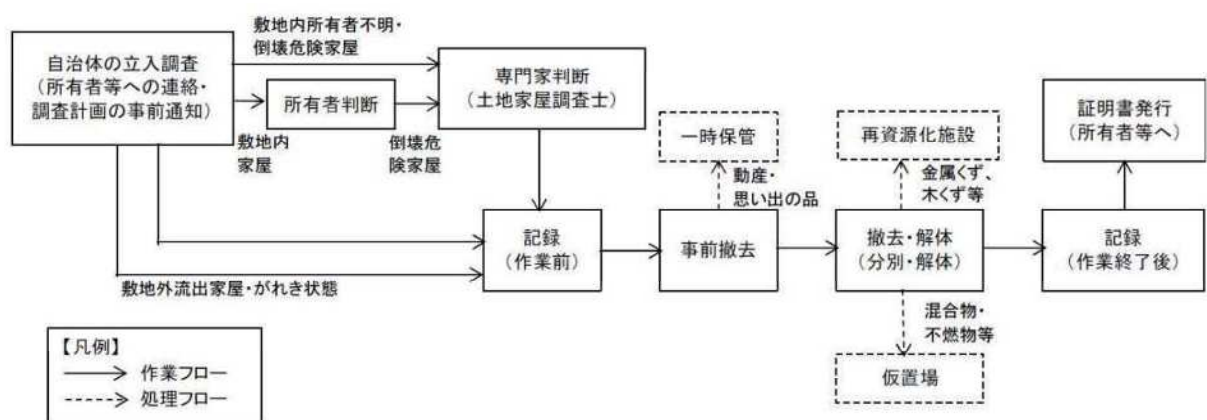
図8 損壊家屋等の作業フロー及び廃棄物処理フロー
