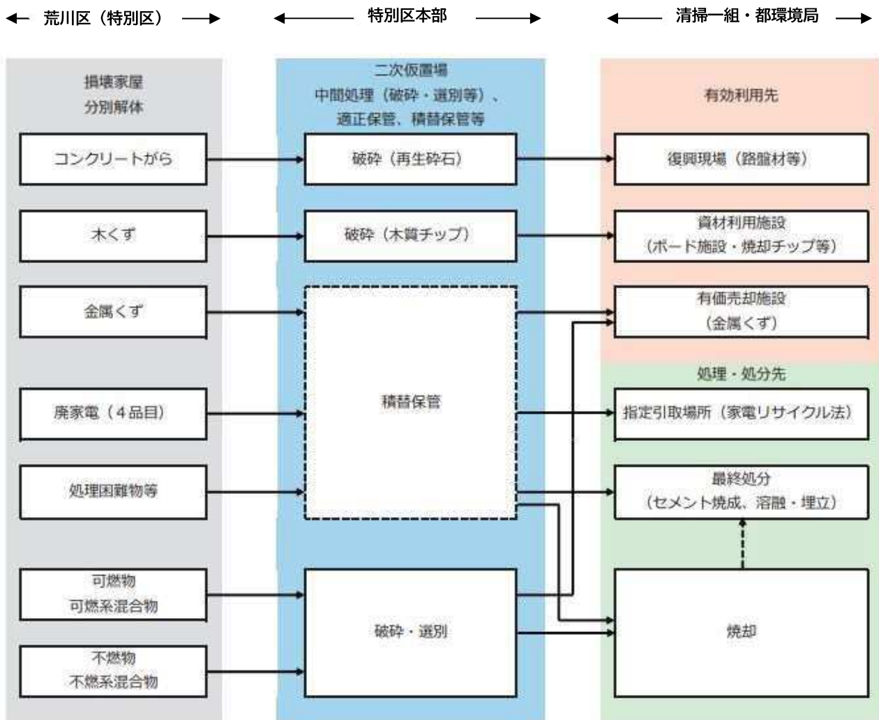
図 3-2 解体廃棄物の標準処理フロー
